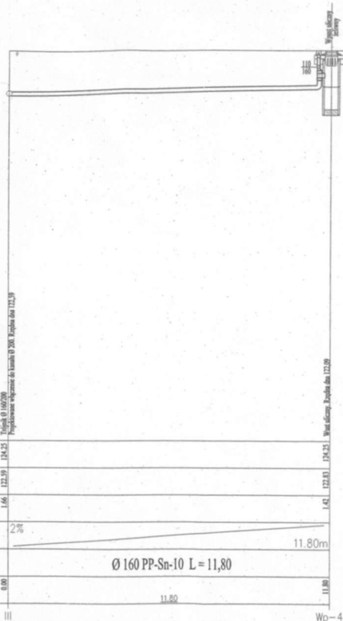
Profil przewodu kanalizacji deszczowej na odcinku od węzła III do Wp-4
