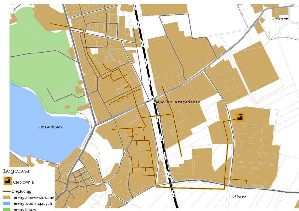
Rysunek 7: Przebieg sieci ciepłowniczej
