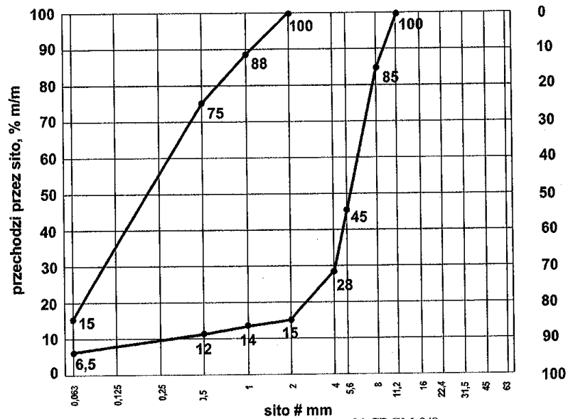
Rys. 5. Uziarnienie mieszanki CBGM 0/8
