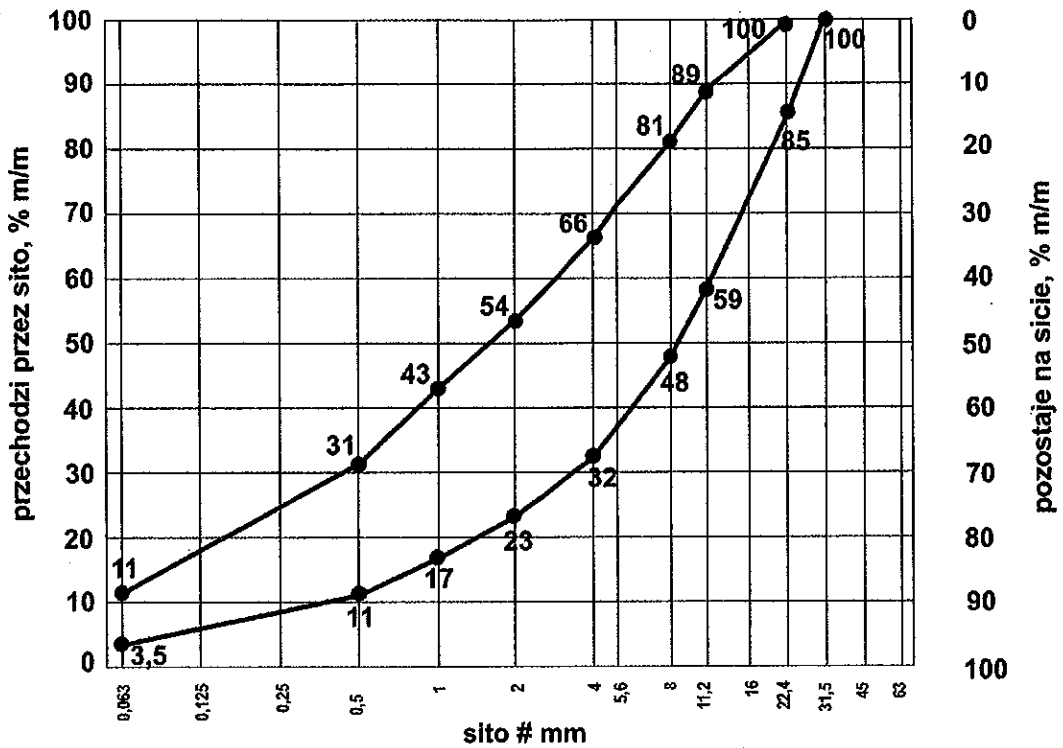
Rys. 2. Uziarnienie mieszanki CBGM 0/22,4
