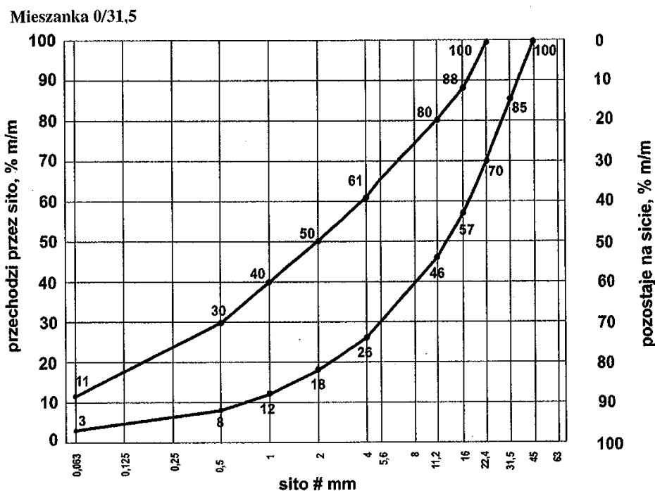
Rys. 1. Uziarnienie mieszanki CBGM 0/31,5
