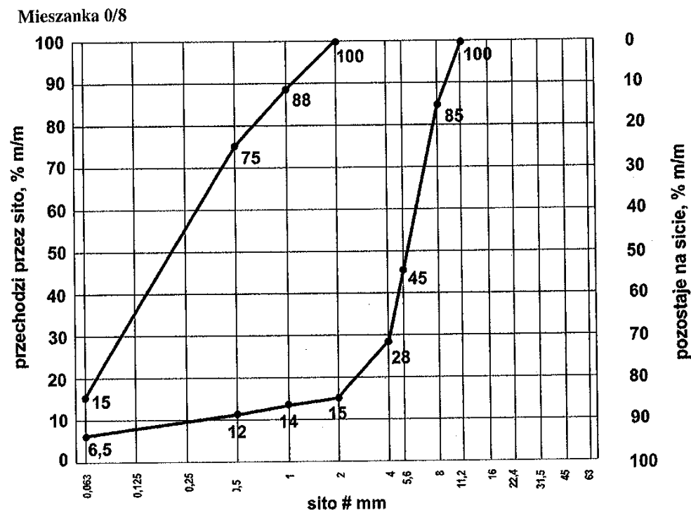
Rys.5. Uziarnienie mieszanki CBGM 0/8
